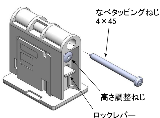
本体(扉側部品)
